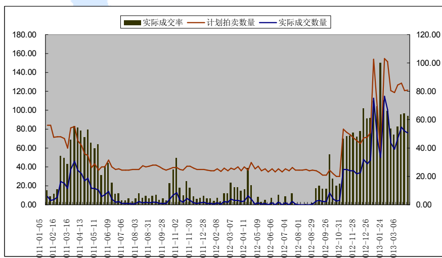
图2 临储小麦拍卖成交情况
