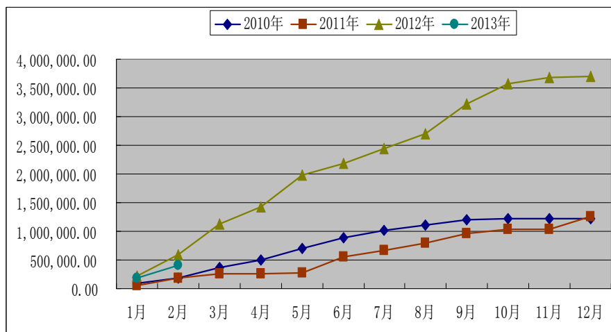
图1 2010年以来小麦进口情况
